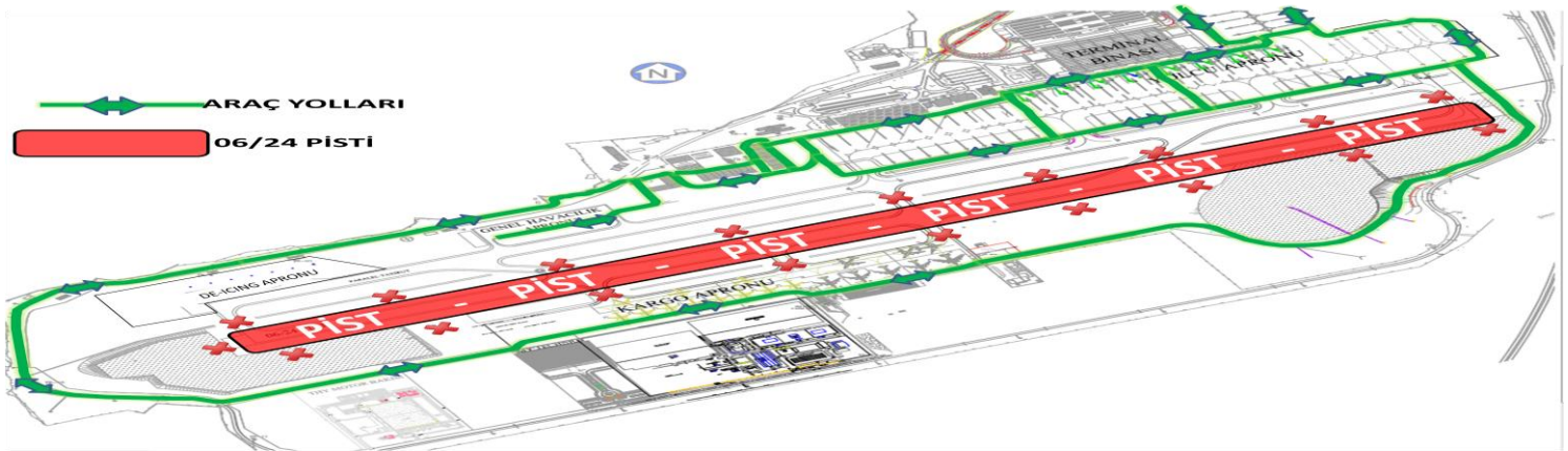
Şekil 1: Sabiha Gökçen Havalimanı Pist ve Araç Yolları
