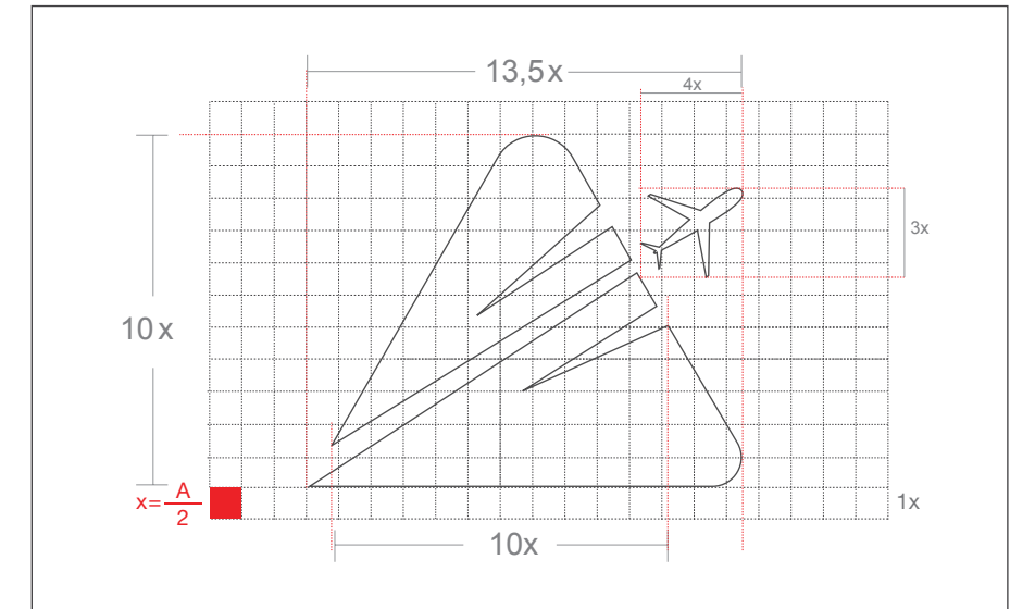
Heaş sembolünün teknik çizimi
